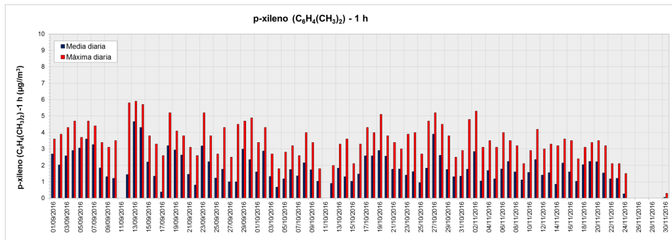
Figura 45. Valores de concentración medios y máximos diarios de p-Xileno (1 h) medidos en el equipo de Paso Abierto (OP2) ubicado en Dock Sud (período septiembre-noviembre 2016). Los resultados se expresan en \mu\text{g} \cdot \text{m}^{-3} .
