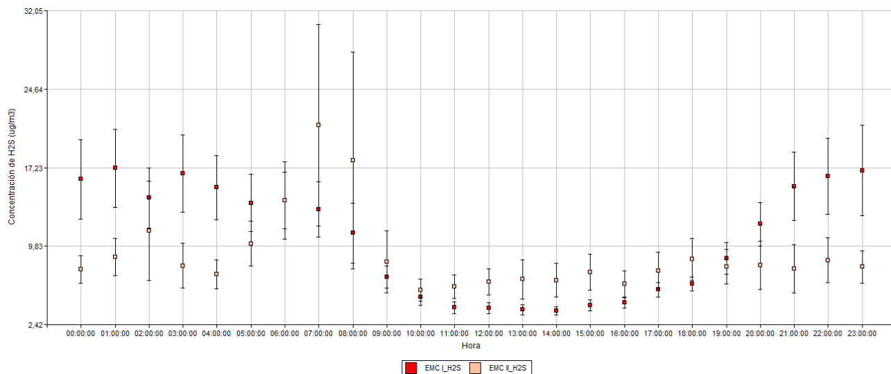
Figura 30. Variación horaria (media \pm error estándar) en la concentración de H_2S medido en la Estación de Monitoreo Continuo Dock Sud (EMC I) y en la Estación de Monitoreo Continuo Lanús (EMC II) para el período septiembre-noviembre 2016. Los resultados se expresan en \mu g.m^{-3} .
