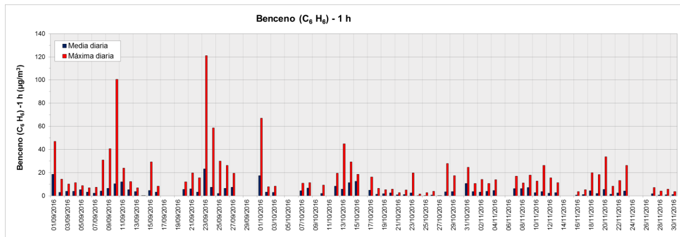
Figura 38. Valores de concentración medios y máximos diarios de benceno (1 h) medidos en el equipo de Paso Abierto (OP1) ubicado en Dock Sud (período septiembre-noviembre 2016). Los resultados se expresan en \mu\text{g}.\text{m}^{-3} .
