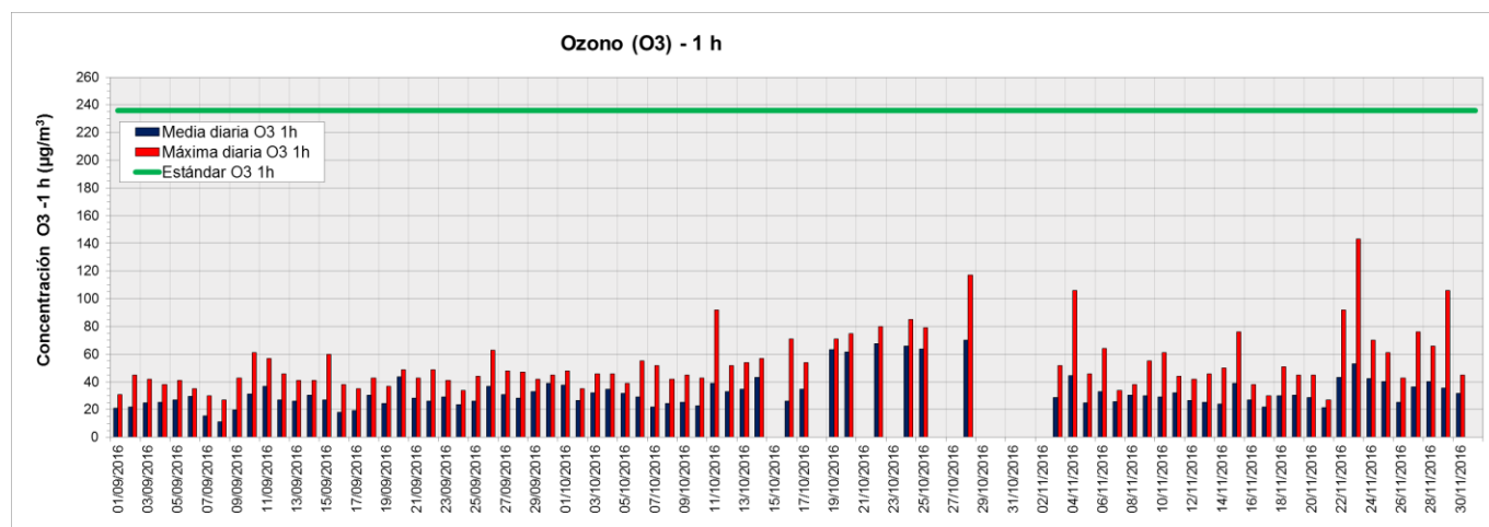
Figura 9. Valores de concentración medios y máximos diarios de O_3 (1 h) medidos en la Estación de Monitoreo Continuo Dock Sud (EMC I) período septiembre-noviembre 2016. Los resultados se expresan en \mu g.m^{-3} .
