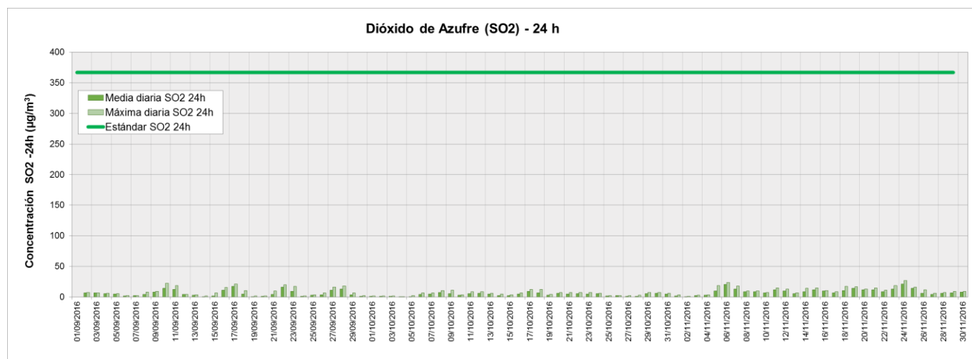
Figura 14. Valores de concentración medios y máximos diarios de SO 2 (24 h) medidos en la Estación de Monitoreo Continuo Lanús (EMC II) período septiembre-noviembre 2016. Los resultados se expresan en \mu\text{g.m}^{-3} .
