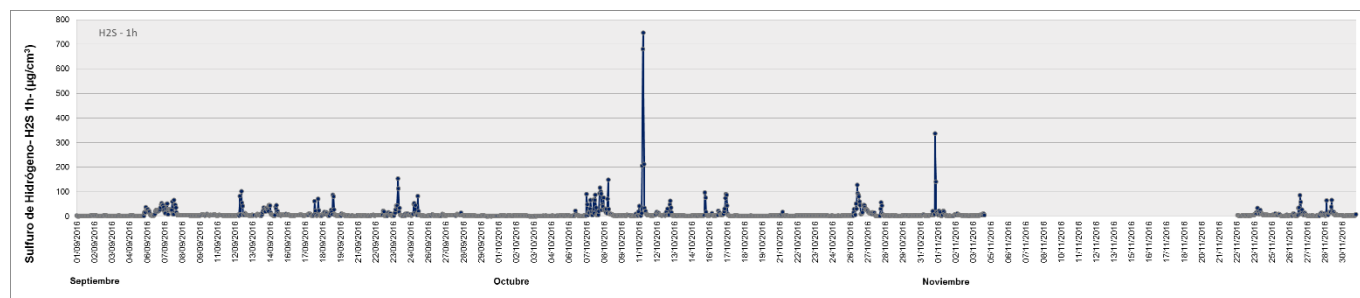
Figura 29. Variación horaria en la concentración de H_2S medida en la Estación de Monitoreo Continuo Lanús (EMC II) para el período septiembre-noviembre 2016. Los resultados se expresan en \mu g.m^{-3} .
