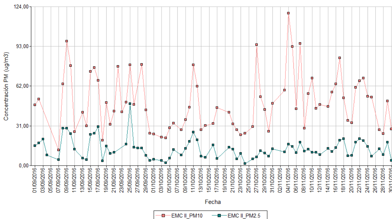
Figura 36. Variación diaria en la concentración de PM 10 y PM 2.5 (24 h) medidos en la Estación de Monitoreo Continuo Lanús (EMC II) para el período septiembre-noviembre 2016. Los resultados se expresan en \mu\text{g}\cdot\text{m}^{-3} .
