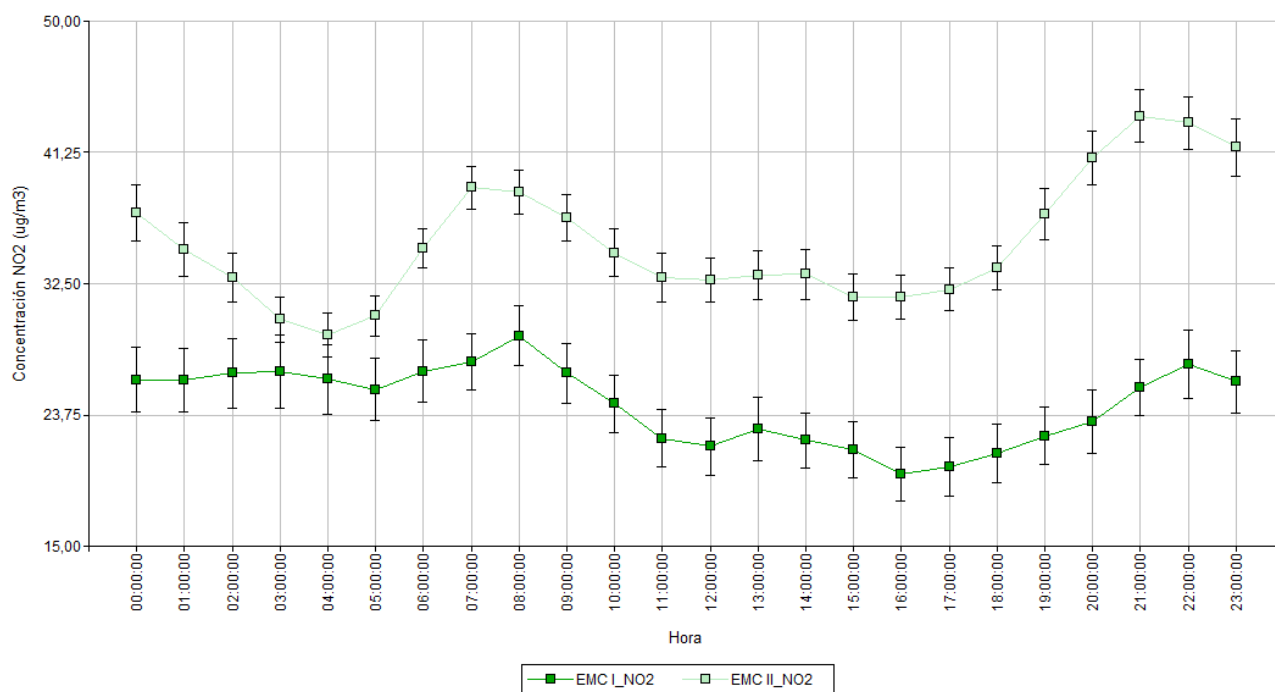
Figura 22. Variación horaria (media \pm error estándar) en la concentración de NO 2 medido en la Estación de Monitoreo Continuo Dock Sud (EMC I) y en la Estación de Monitoreo Continuo Lanús (EMC II) para el período septiembre-noviembre 2016. Los resultados se expresan en \mu\text{g}\cdot\text{m}^{-3} .
