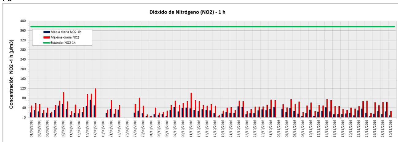
Figura 7. Valores de concentración medios y máximos diarios de NO 2 (1 h) medidos en la Estación de Monitoreo Continuo Dock Sud (EMC I) período septiembre-noviembre 2016. Los resultados se expresan en \mu\text{g}.\text{m}^{-3} .
