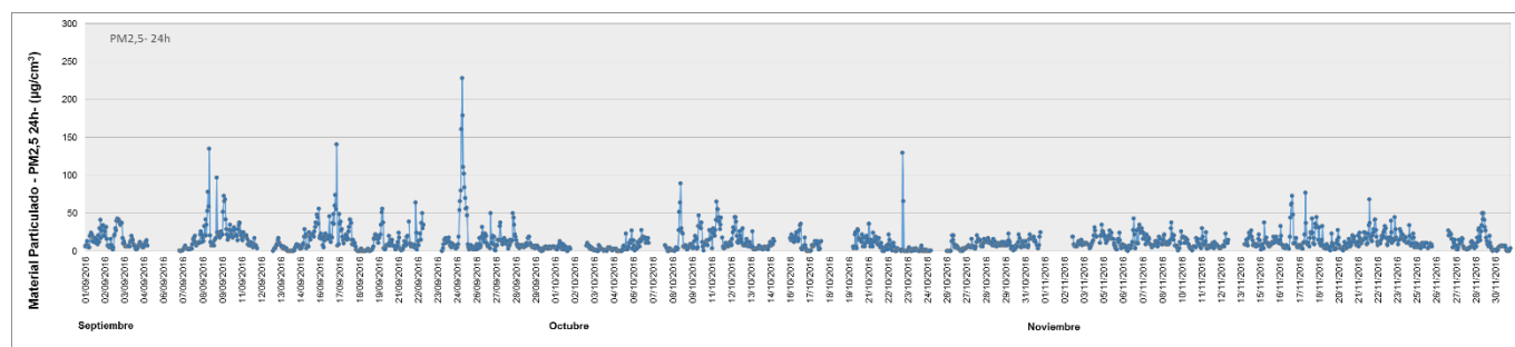
Figura 34. Variación horaria en la concentración de PM 2.5 medida en la Estación de Monitoreo Continuo Lanús (EMC II) para el período septiembre-noviembre 2016. Los resultados se expresan en \mu\text{g}\cdot\text{m}^{-3} .
