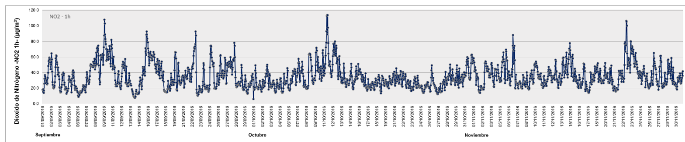
Figura 21. Variación horaria en la concentración de NO 2 medida en la Estación de Monitoreo Continuo Lanús (EMC II) para el período septiembre-noviembre 2016. Los resultados se expresan en \mu\text{g}\cdot\text{m}^{-3} .
