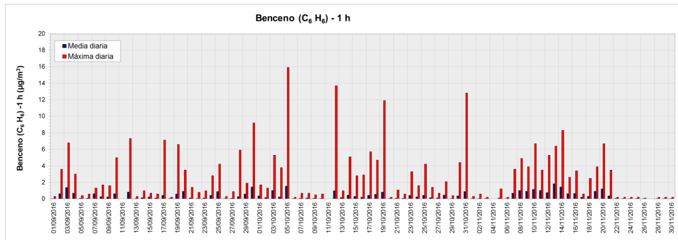
Figura 39. Valores de concentración medios y máximos diarios de benceno (1 h) medidos en el equipo de Paso Abierto (OP2) ubicado en Dock Sud (período septiembre-noviembre 2016). Los resultados se expresan en \mu\text{g} \cdot \text{m}^{-3} .
