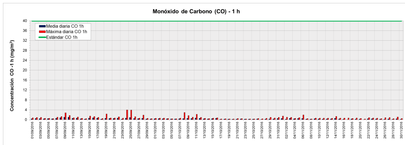
Figura 4. Valores de concentración medios y máximos diarios de CO (1 h) medidos en la Estación de Monitoreo Continuo Lanús (EMC II) período septiembre-noviembre 2016. Los resultados se expresan en \text{mg.m}^{-3} .
