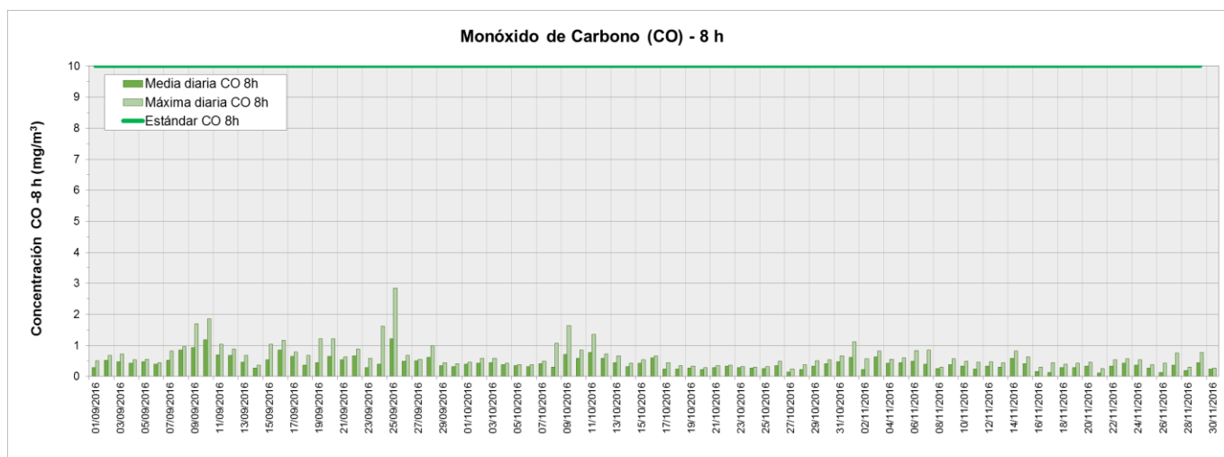
Figura 6. Valores de concentración medios y máximos diarios de CO (8 h) medidos en la Estación de Monitoreo Continuo Lanús (EMC II) período septiembre-noviembre 2016. Los resultados se expresan en \text{mg.m}^{-3} .
