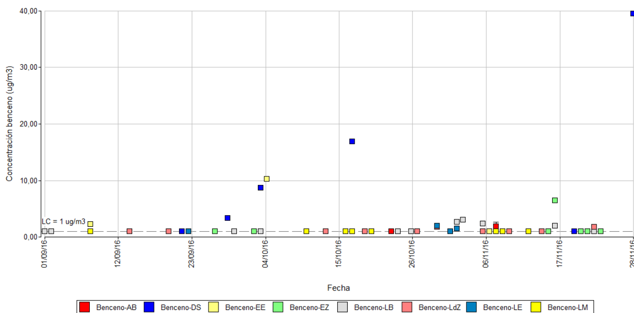
Figura 52. Concentración de benceno ( C_6H_6 – 40 min) medida en las ocho áreas de estudio en los meses de septiembre-noviembre 2016. Los resultados se expresan en \mu g/m^3 . LC: Límite de Cuantificación.
