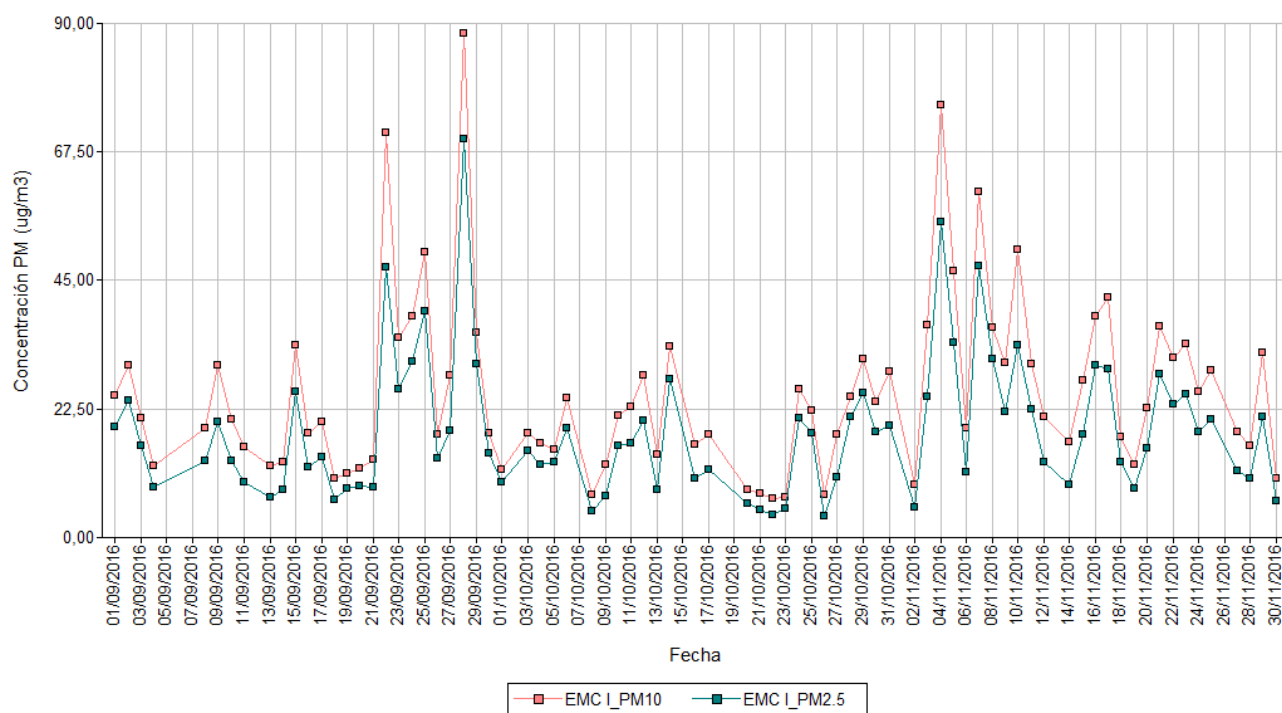
Figura 35. Variación diaria en la concentración de PM 10 y PM 2.5 (24 h) medidos en la Estación de Monitoreo Continuo Dock Sud (EMC I) para el período septiembre-noviembre 2016. Los resultados se expresan en \mu\text{g}\cdot\text{m}^{-3} .
