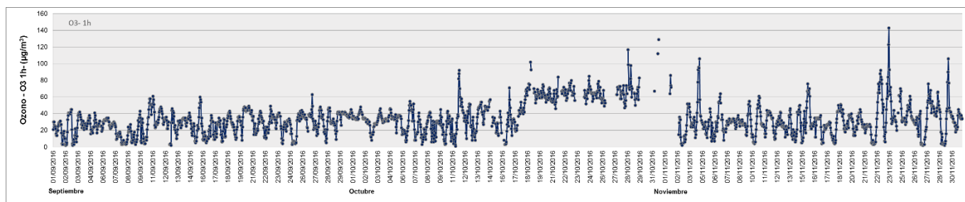
Figura 23. Variación horaria en la concentración de O 3 medida en la Estación de Monitoreo Continuo Dock Sud (EMC I) para el período septiembre-noviembre 2016. Los resultados se expresan en \mu\text{g}\cdot\text{m}^{-3} .
