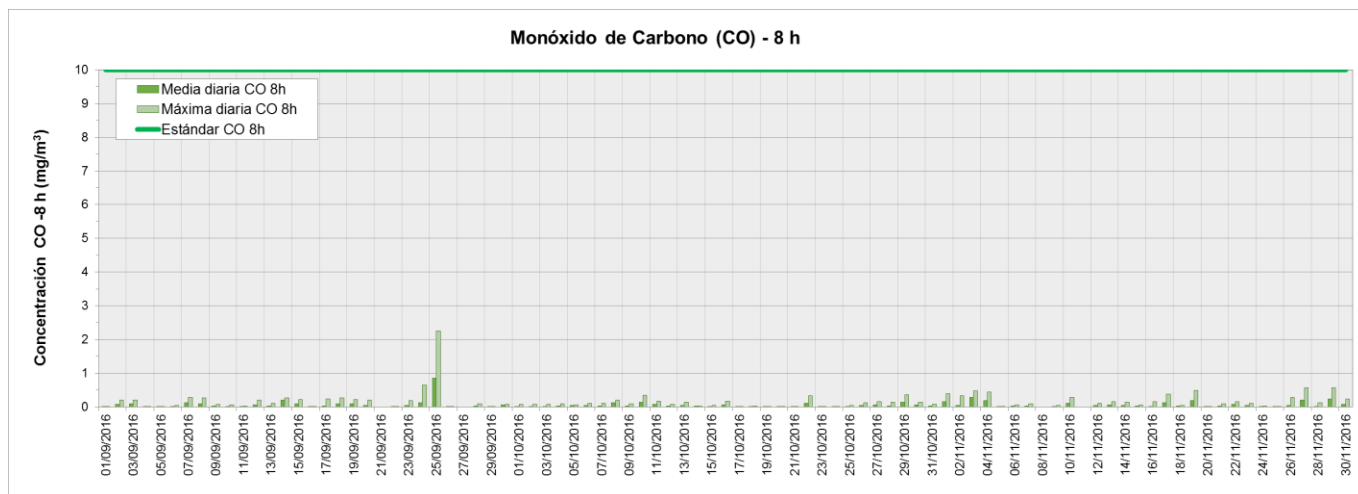
Figura 5. Valores de concentración medios y máximos diarios de CO (8 h) medidos en la Estación de Monitoreo Continuo Dock Sud (EMC I) período septiembre-noviembre 2016. Los resultados se expresan en \text{mg.m}^{-3} .
