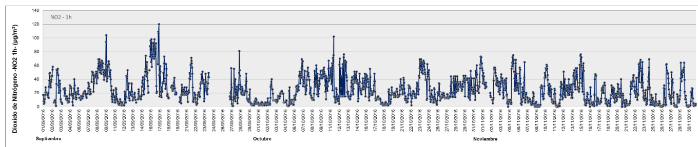
Figura 20. Variación horaria en la concentración de NO 2 medida en la Estación de Monitoreo Continuo Dock Sud (EMC I) para el período septiembre-noviembre 2016. Los resultados se expresan en \mu\text{g}\cdot\text{m}^{-3} .
