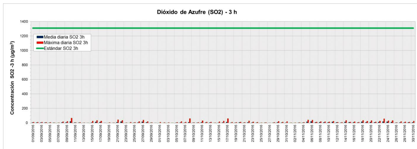
Figura 12. Valores de concentración medios y máximos diarios de SO 2 (3 h) medidos en la Estación de Monitoreo Continuo Lanús (EMC II) período septiembre-noviembre 2016. Los resultados se expresan en \mu\text{g.m}^{-3} .
