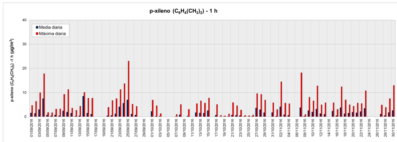
Figura 44. Valores de concentración medios y máximos diarios de p-Xileno (1 h) medidos en el equipo de Paso Abierto (OP1) ubicado en Dock Sud (período septiembre-noviembre 2016). Los resultados se expresan en \mu\text{g} \cdot \text{m}^{-3} .
