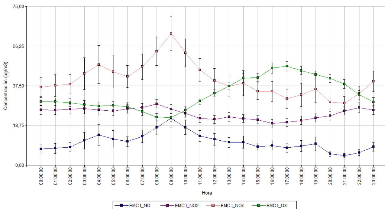
Figura 24. Variación horaria (media \pm error estándar) en la concentración de NO x , NO 2 , NO y O 3 medidos en la EMC I en Dock Sud para el período septiembre-noviembre 2016. Los resultados se expresan en \mu\text{g}\cdot\text{m}^{-3} .
