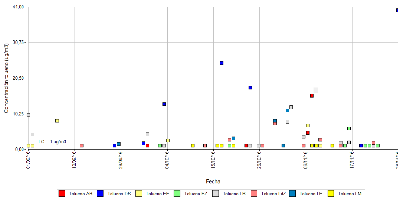
Figura 53. Concentración de tolueno ( C_6H_5CH_3 - 40 min) medida en las ocho áreas de estudio en los meses de septiembre-noviembre 2016. Los resultados se expresan en \mu g/m^3 . LC: Límite de Cuantificación.
