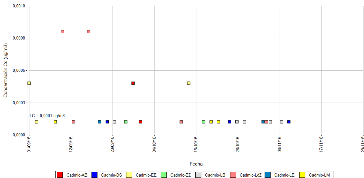
Figura 50. Concentración de cadmio en PM10 24 horas (Cd - 24 h) medida en las ocho áreas de estudio en los meses de septiembre-noviembre 2016. Los resultados se expresan en \mu\text{g}/\text{m}^3 . LC: Límite de Cuantificación.
