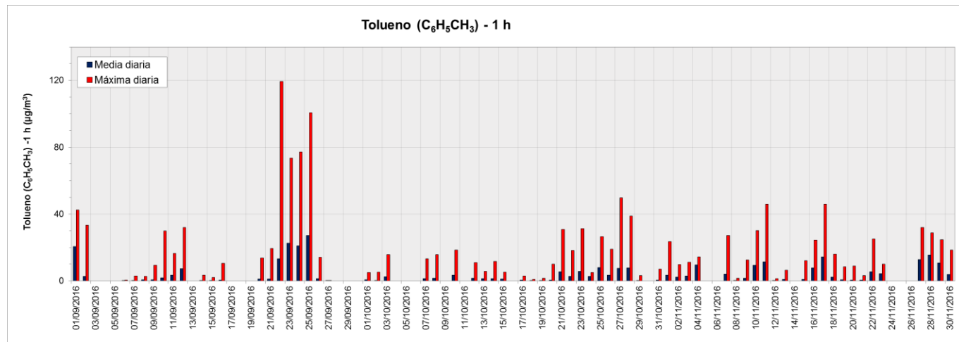
Figura 40. Valores de concentración medios y máximos diarios de tolueno (1 h) medidos en el equipo de Paso Abierto (OP1) ubicado en Dock Sud (período septiembre-noviembre 2016). Los resultados se expresan en \mu\text{g} \cdot \text{m}^{-3} .
