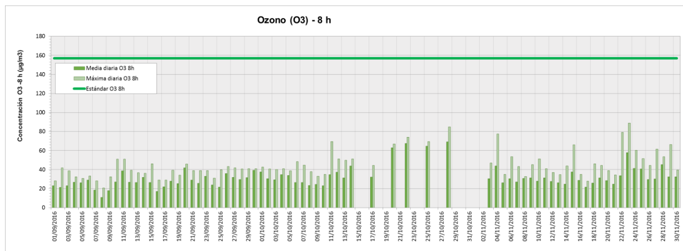
Figura 10. Valores de concentración medios y máximos diarios de O_3 (8 h) medidos en la Estación de Monitoreo Continuo Dock Sud (EMC I) período septiembre-noviembre 2016. Los resultados se expresan en \mu g.m^{-3} .
