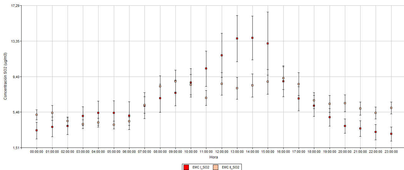
Figura 27. Variación horaria (media \pm error estándar) en la concentración de SO 2 medido en la EMC I en Dock Sud y en la EMC II en Lanús para el período septiembre-noviembre 2016. Los resultados se expresan en \mu\text{g} \cdot \text{m}^{-3} .
