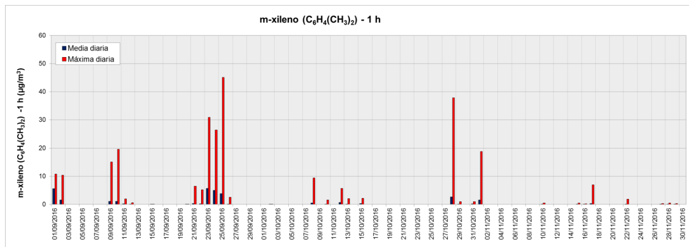
Figura 42. Valores de concentración medios y máximos diarios de m-xileno (1 h) medidos en el equipo de Paso Abierto (OP1) ubicado en Dock Sud (período septiembre-noviembre 2016). Los resultados se expresan en \mu\text{g}.\text{m}^{-3} .
