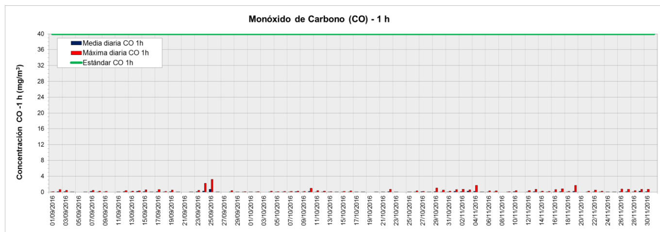
Figura 3. Valores de concentración medios y máximos diarios de CO (1 h) medidos en la Estación de Monitoreo Continuo Dock Sud (EMC I) período septiembre-noviembre 2016. Los resultados se expresan en \text{mg.m}^{-3} .
