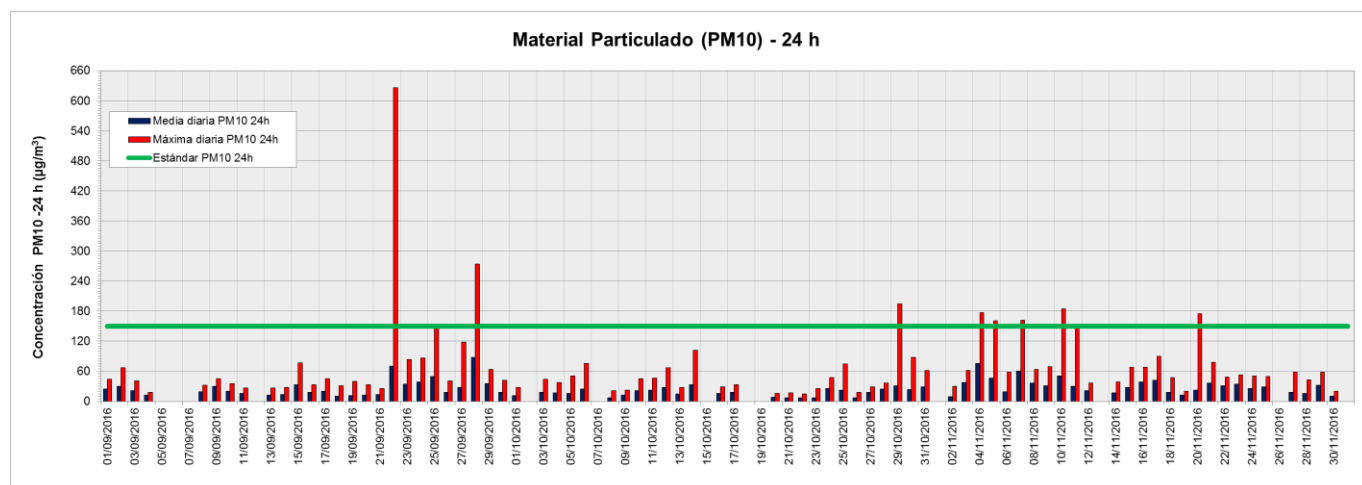
Figura 15. Valores de concentración medios y máximos de PM 10 (24 h) medidos en la Estación de Monitoreo Continuo Dock Sud (EMC I) período septiembre-noviembre 2016. Los resultados se expresan en \mu\text{g}\cdot\text{m}^{-3} .
