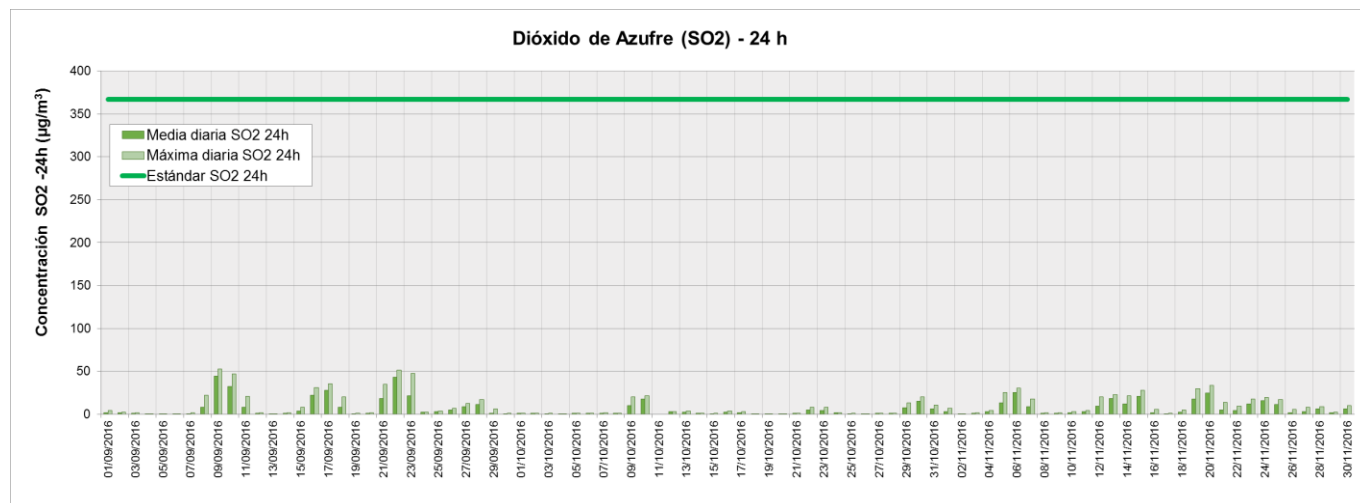
Figura 13. Valores de concentración medios y máximos diarios de SO 2 (24 h) medidos en la Estación de Monitoreo Continuo Dock Sud (EMC I) período septiembre-noviembre 2016. Los resultados se expresan en \mu\text{g.m}^{-3} .
