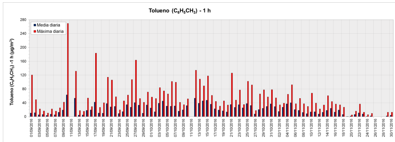
Figura 41. Valores de concentración medios y máximos diarios de tolueno (1 h) medidos en el equipo de Paso Abierto (OP2) ubicado en Dock Sud (período septiembre-noviembre 2016). Los resultados se expresan en \mu\text{g} \cdot \text{m}^{-3} .
