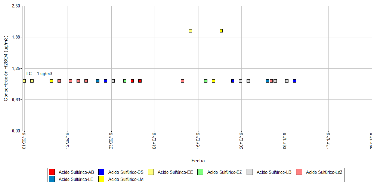
Figura 51. Concentración de ácido sulfúrico en PM2.5 24 horas ( \text{H}_2\text{SO}_4 - 24 h) medida en las ocho áreas de estudio en los meses de septiembre-noviembre 2016. Los resultados se expresan en \mu\text{g}/\text{m}^3 . LC: Límite de Cuantificación.
