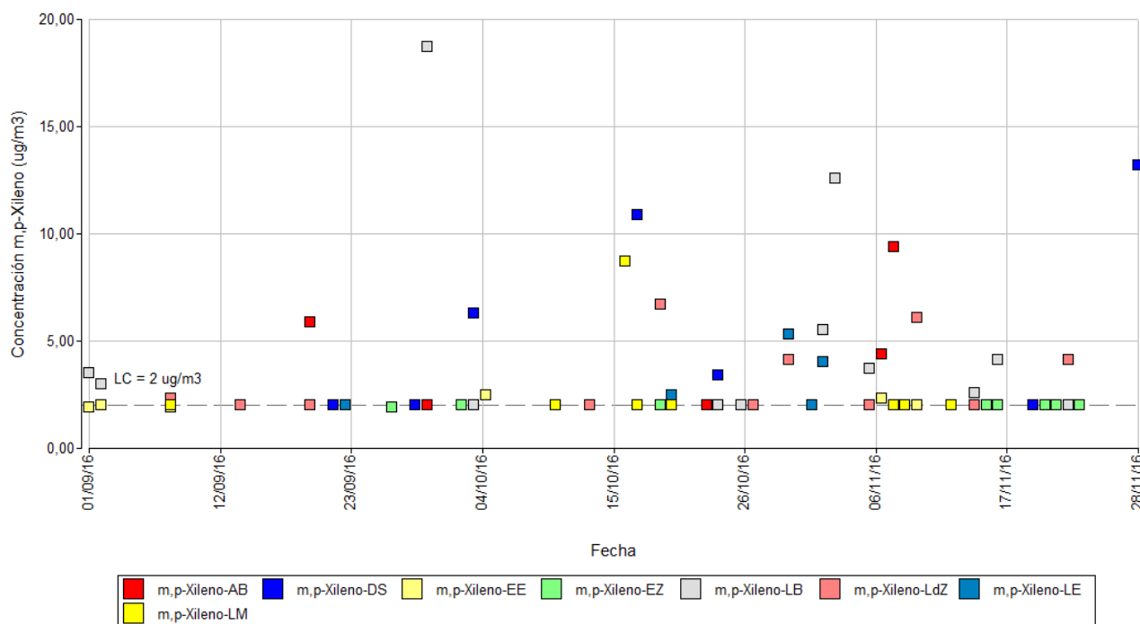
Figura 54. Concentración de m,p-xileno ( C_6H_4(CH_3)_2 - 40 min) medida en las ocho áreas de estudio en los meses de septiembre-noviembre 2016. Los resultados se expresan en \mu g/m^3 . LC: Límite de Cuantificación.
