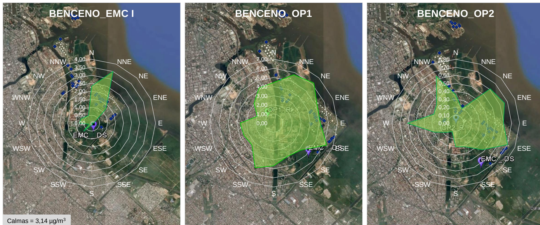
Figura 47. Rosas de contaminantes para Benceno medido en la EMC I, OP1 y OP2 en Dock Sud en los meses de septiembre-noviembre 2016. Se presentan los valores promedio de concentración de benceno ( \mu\text{g}/\text{m}^3 ) para las 16 direcciones de viento.
