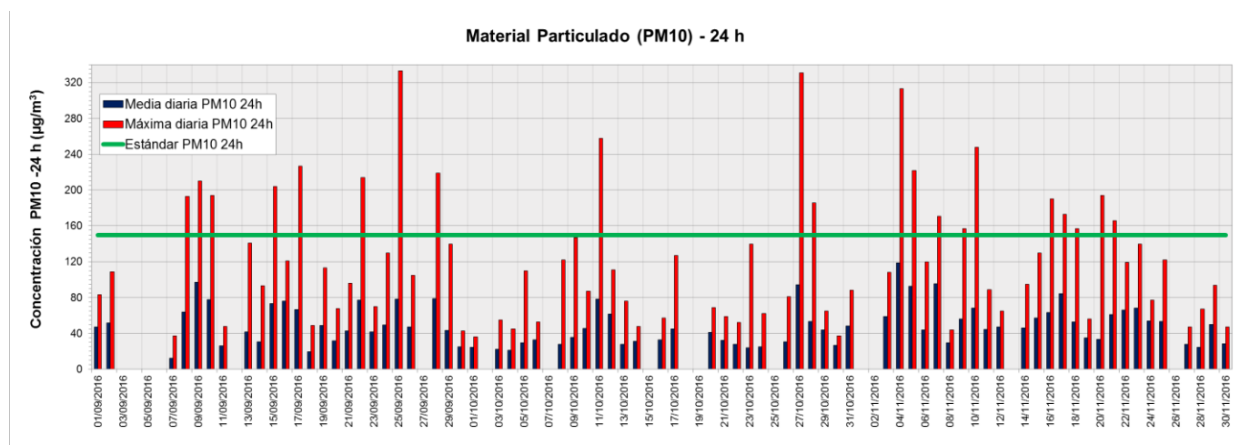
Figura 16. Valores de concentración medios y máximos de PM 10 (24 h) medidos en la Estación de Monitoreo Continuo Lanús (EMC II) período septiembre-noviembre 2016. Los resultados se expresan en \mu\text{g}\cdot\text{m}^{-3} .
