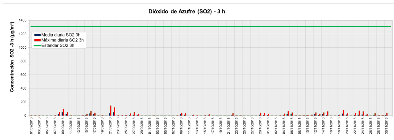
Figura 11. Valores de concentración medios y máximos diarios de SO 2 (3 h) medidos en la Estación de Monitoreo Continuo Dock Sud (EMC I) período septiembre-noviembre 2016. Los resultados se expresan en \mu\text{g} \cdot \text{m}^{-3} .
