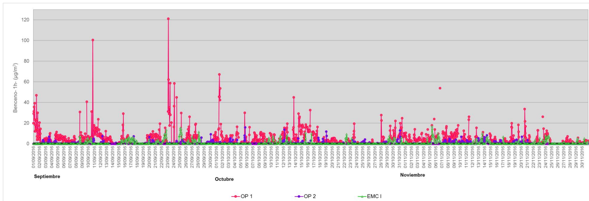
Figura 46. Variación horaria en la concentración de Benceno medida con los Open Path 1 y 2 y la EMC I para el período septiembre-noviembre 2016. Los resultados se expresan en \mu\text{g}\cdot\text{m}^{-3} .
