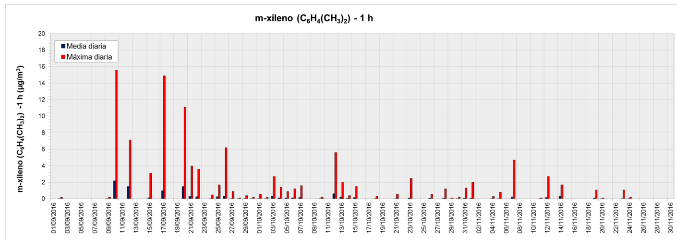
Figura 43. Valores de concentración medios y máximos diarios de m-Xileno (1 h) medidos en el equipo de Paso Abierto (OP2) ubicado en Dock Sud (período septiembre-noviembre 2016). Los resultados se expresan en \mu\text{g}.\text{m}^{-3} .
