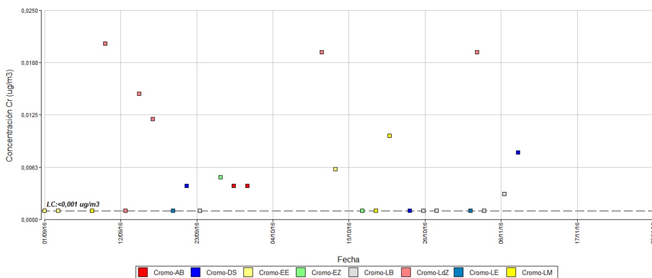
Figura 49. Concentración de cromo total en PM10 24 horas (Cr - 24 h) medida en las ocho áreas de estudio en los meses de septiembre-noviembre 2016. Los resultados se expresan en \mu\text{g}/\text{m}^3 . LC: Límite de Cuantificación.
