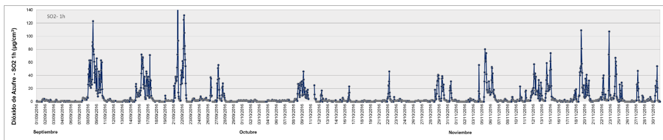
Figura 25. Variación horaria en la concentración de SO 2 medida en la Estación de Monitoreo Continuo Dock Sud (EMC I) para el período septiembre-noviembre 2016. Los resultados se expresan en \mu\text{g} \cdot \text{m}^{-3} .
