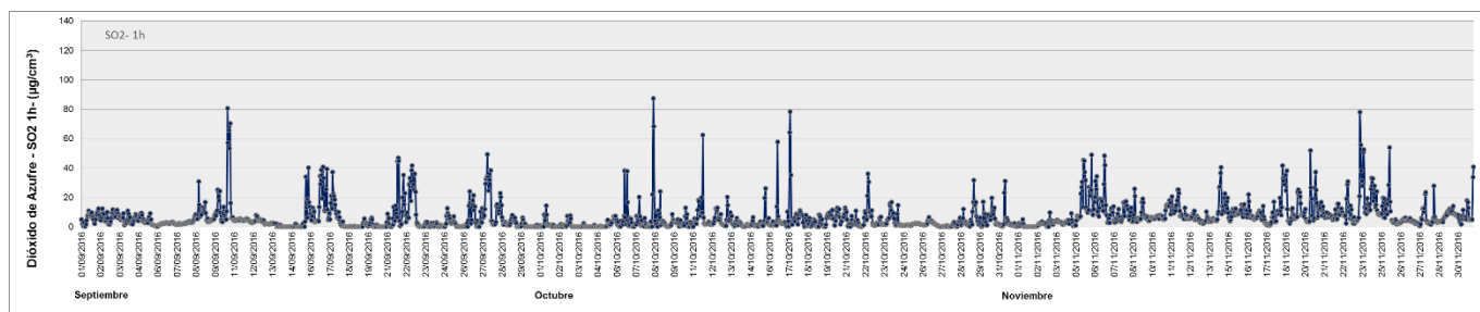
Figura 26. Variación horaria en la concentración de SO 2 medida en la Estación de Monitoreo Continuo Lanús (EMC II) para el período septiembre-noviembre 2016. Los resultados se expresan en \mu\text{g} \cdot \text{m}^{-3} .
