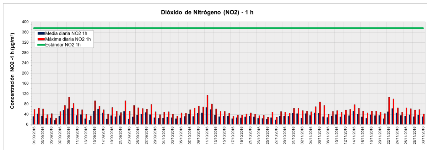
Figura 8. Valores de concentración medios y máximos diarios de NO 2 (1 h) medidos en la Estación de Monitoreo Continuo Lanús (EMC II) período septiembre-noviembre 2016. Los resultados se expresan en µg.m -3 .
