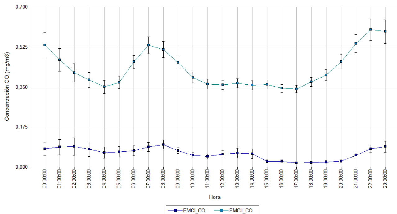
Figura 19. Variación horaria (media \pm error estándar) en la concentración de CO medido en la Estación de Monitoreo Continuo Dock Sud (EMC I) y en la Estación de Monitoreo Continuo Lanús (EMC II) para el período septiembre-noviembre 2016. Los resultados se expresan en \text{mg.m}^{-3} .
