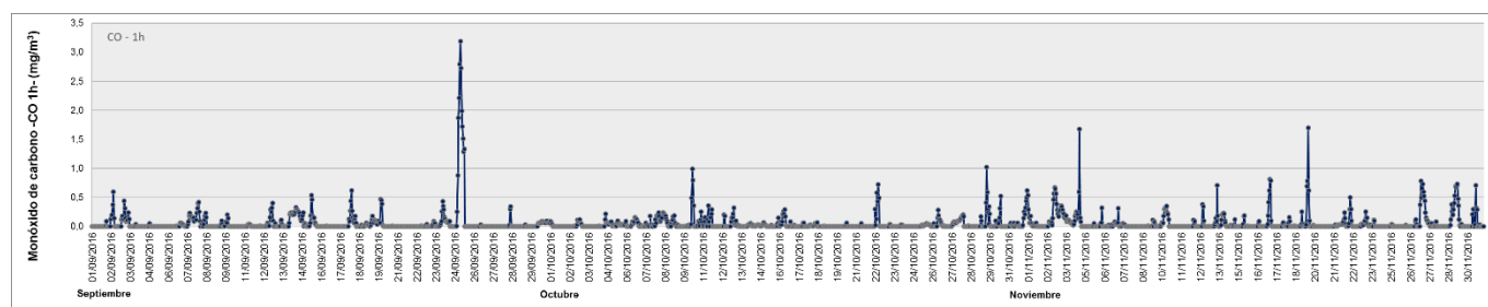
Figura 17. Variación horaria en la concentración de CO medida en la Estación de Monitoreo Continuo Dock Sud (EMC I) para el período septiembre-noviembre 2016. Los resultados se expresan en mg.m -3 .
