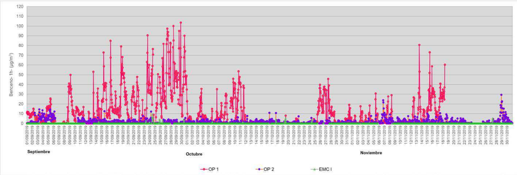
Figura 55. Variación horaria en la concentración de Benceno medida con los Open Path 1 y 2 y la EMC I para el período septiembre - noviembre 2019. Los resultados se expresan en \mu\text{g}\cdot\text{m}^{-3} .
