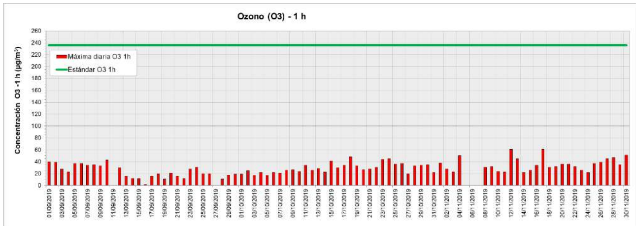
Figura 14. Valores de concentración máximos diarios de O 3 (1 h) medidos en la Estación de Monitoreo Continuo Dock Sud (EMC I) período septiembre - noviembre 2019. Los resultados se expresan en µg.m -3 .
