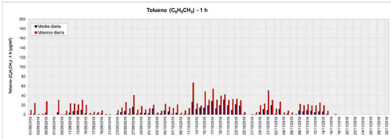
Figura 49. Valores de concentración medios y máximos diarios de tolueno (1 h) medidos en el equipo Open Path (OP1) ubicado en Dock Sud (período septiembre - noviembre 2019). Los resultados se expresan en \mu\text{g}.\text{m}^{-3}
