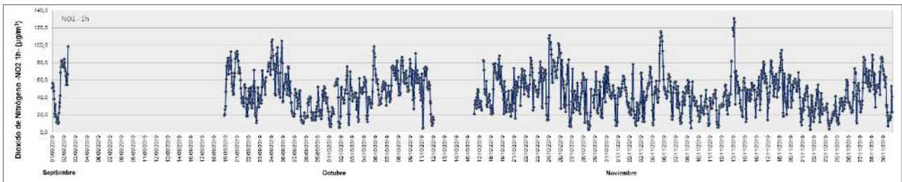
Figura 29. Variación horaria en la concentración de NO 2 medida en la Estación de Monitoreo Continuo La Boca para el período septiembre - noviembre 2019. Los resultados se expresan en µg.m -3 .
