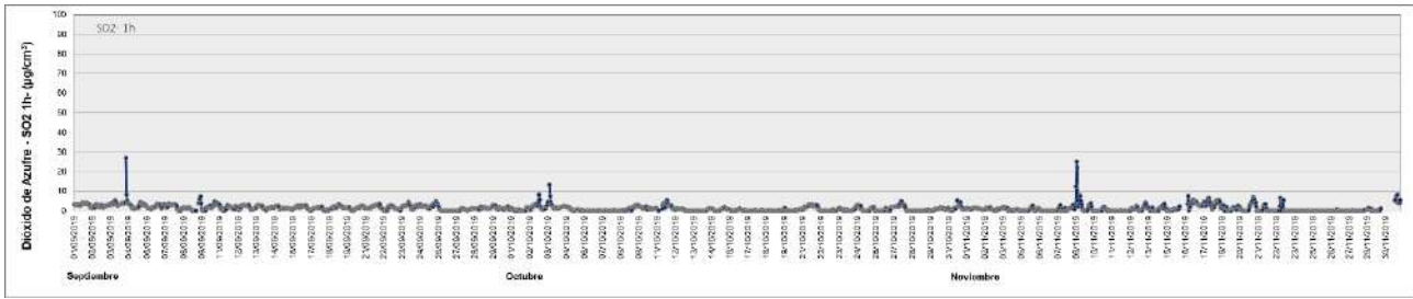
Figura 33. Variación horaria en la concentración de SO 2 medida en la Estación de Monitoreo Continuo La Matanza (EMC II) para el período septiembre - noviembre 2019. Los resultados se expresan en µg.m -3 .
