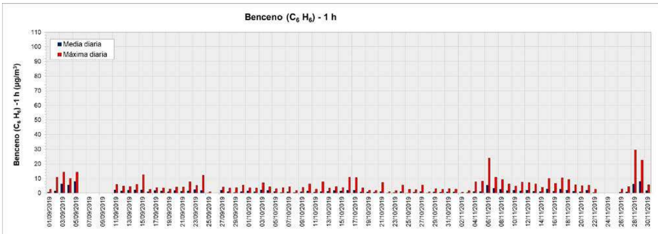
Figura 48. Valores de concentración medios y máximos diarios de benceno (1 h) medidos en el equipo Open Path (OP2) ubicado en Dock Sud (período septiembre - noviembre 2019). Los resultados se expresan en \mu\text{g}\cdot\text{m}^{-3} .
