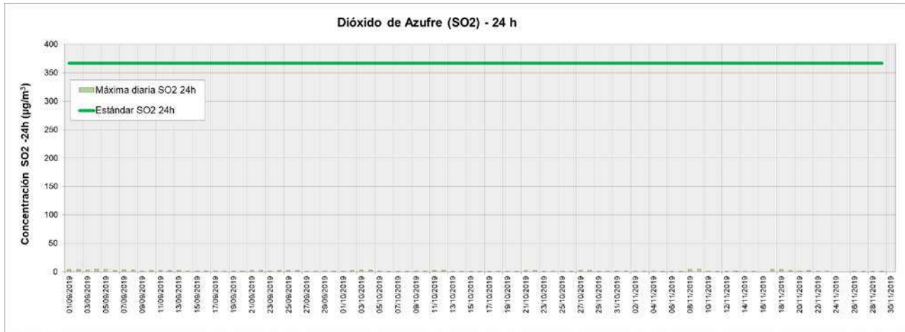
Figura 19. Valores de concentración máximos diarios de SO 2 (24 h) medidos en la Estación de Monitoreo Continuo La Matanza (EMC II) período septiembre - noviembre 2019. Los resultados se expresan en µg.m -3 .
