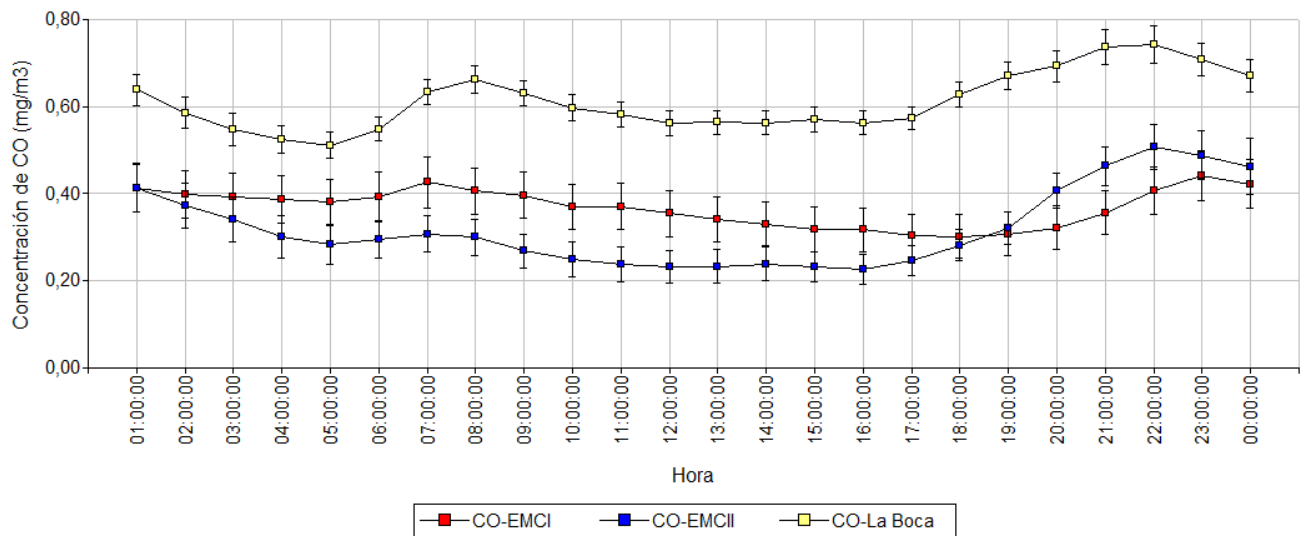
Figura 26. Variación horaria (media \pm error estándar) en la concentración de CO medido en las Estaciones de Monitoreo Continuo de Dock Sud (EMC I), La Matanza (EMC II) y La Boca para el período septiembre - noviembre 2019. Los resultados se expresan en \text{mg}\cdot\text{m}^{-3} .
