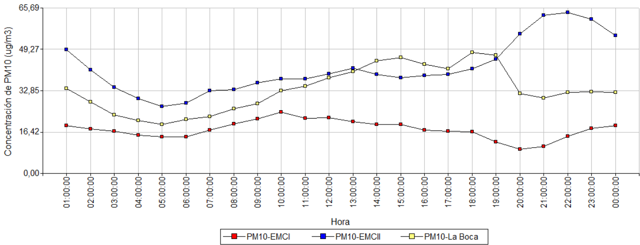
Figura 45. Variación horaria en la concentración de PM 10 medidos en la Estación de Monitoreo Continuo de Dock Sud (EMC I), La Matanza (EMC II) y La Boca para el período septiembre - noviembre 2019. Los resultados se expresan en \mu\text{g}\cdot\text{m}^{-3} .
