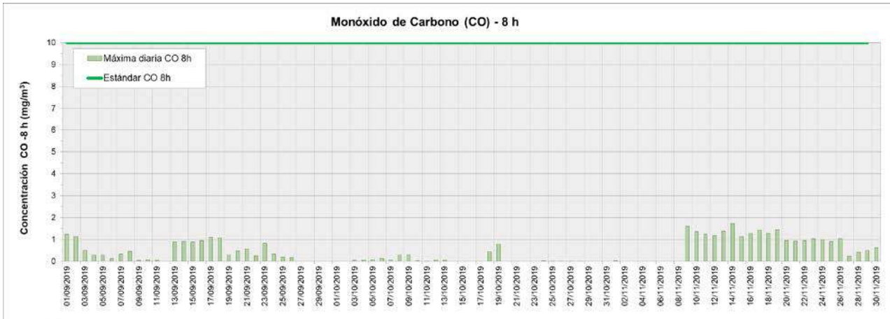
Figura 9. Valores de concentración máximos diarios de CO (8 h) medidos en la Estación de Monitoreo Continuo La Matanza (EMC II) período septiembre - noviembre 2019. Los resultados se expresan en \text{mg}\cdot\text{m}^{-3} .
