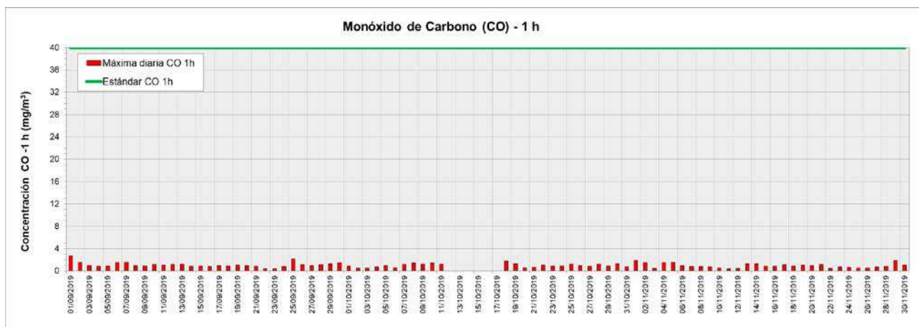
Figura 7. Valores de concentración máximos diarios de CO (1 h) medidos en la Estación de Monitoreo Continuo La Boca período septiembre - noviembre 2019. Los resultados se expresan en \text{mg}\cdot\text{m}^{-3} .
