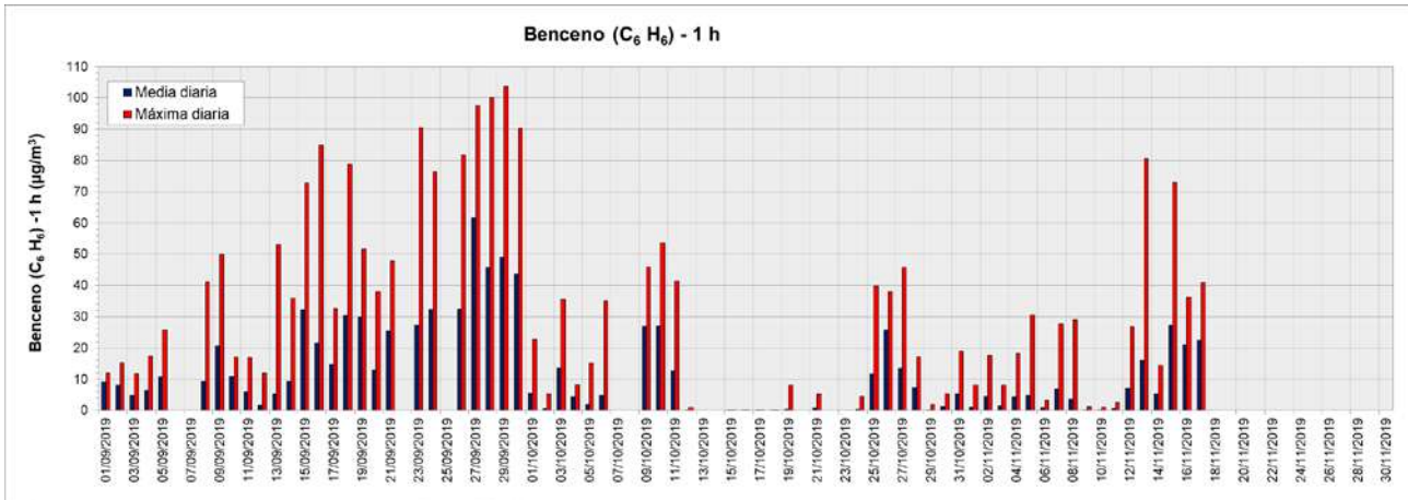
Figura 47. Valores de concentración medios y máximos diarios de benceno (1 h) medidos en el equipo Open Path (OP1) ubicado en Dock Sud (período septiembre - noviembre 2019). Los resultados se expresan en \mu\text{g}\cdot\text{m}^{-3} .
