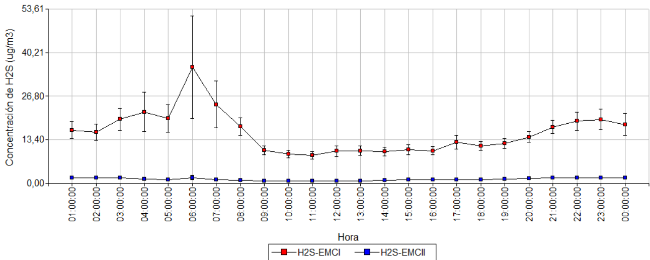
Figura 37. Variación horaria (media \pm error estándar) en la concentración de \text{H}_2\text{S} medido en la Estación de Monitoreo Continuo Dock Sud (EMC I) y en la Estación de Monitoreo Continuo La Matanza (EMC II) para el período septiembre - noviembre 2019. Los resultados se expresan en \mu\text{g}\cdot\text{m}^{-3} .
