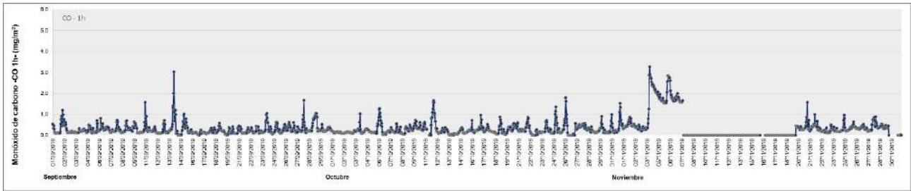
Figura 24. Variación horaria en la concentración de CO medida en la Estación de Monitoreo Continuo La Matanza (EMC II) para el período septiembre - noviembre 2019. Los resultados se expresan en \text{mg}\cdot\text{m}^{-3} .
