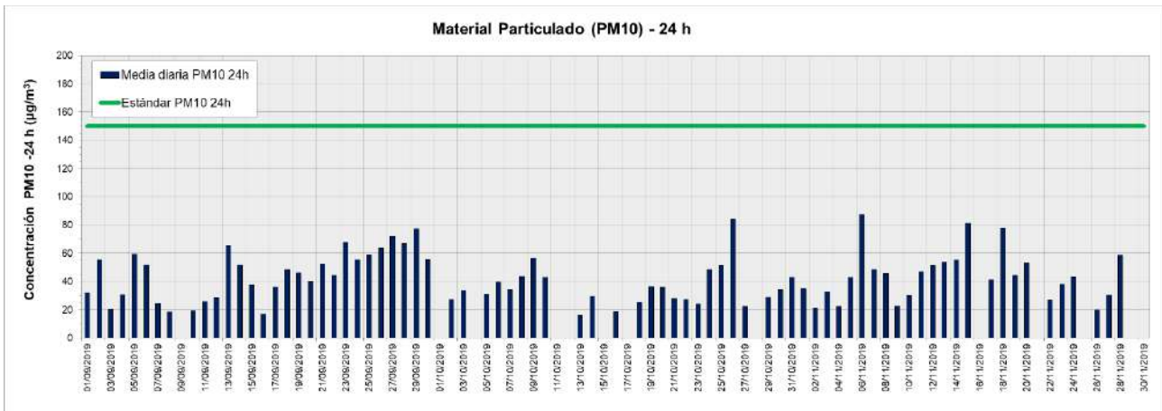
Figura 22. Valores de concentración medios de PM 10 (24 h) medidos en la Estación de Monitoreo Continuo La Boca período septiembre - noviembre 2019. Los resultados se expresan en \mu\text{g}\cdot\text{m}^{-3} .
