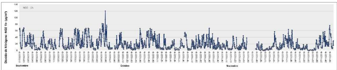
Figura 27. Variación horaria en la concentración de NO 2 medida en la Estación de Monitoreo Continuo Dock Sud (EMC I) para el período septiembre - noviembre 2019. Los resultados se expresan en µg.m -3 .
