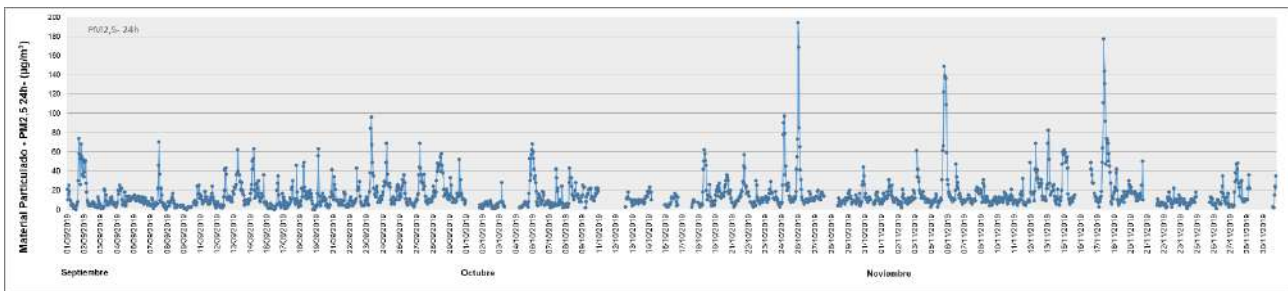
Figura 42. Variación horaria en la concentración de PM2.5 medida en la Estación de Monitoreo Continuo La Matanza (EMC II) para el período septiembre - noviembre 2019. Los resultados se expresan en \mu\text{g.m}^{-3} .
