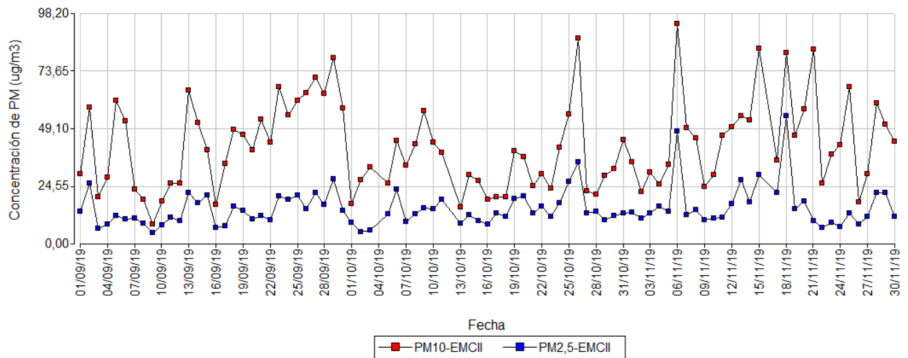
Figura 44. Variación diaria en la concentración de PM 10 y PM 2.5 (24 h) medidos en la Estación de Monitoreo Continuo La Matanza (EMC II) para el período septiembre - noviembre 2019. Los resultados se expresan en \mu\text{g}\cdot\text{m}^{-3} .
