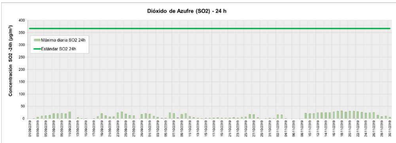
Figura 18. Valores de concentración máximos diarios de SO 2 (24 h) medidos en la Estación de Monitoreo Continuo Dock Sud (EMC I) período septiembre - noviembre 2019. Los resultados se expresan en µg.m -3 .
