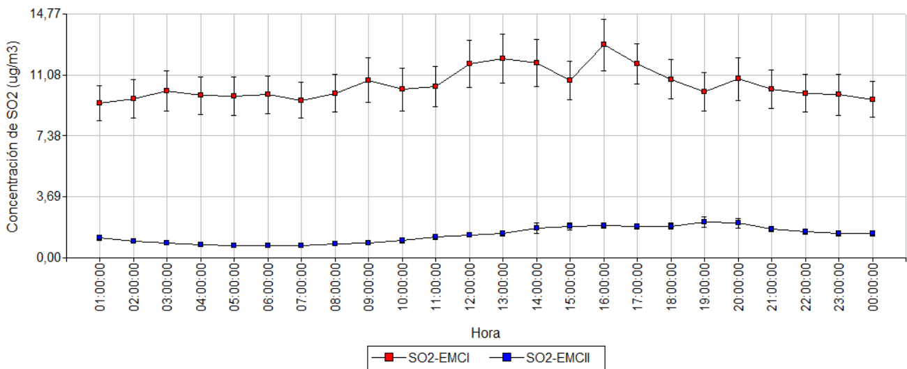
Figura 34. Variación horaria (media ± error estándar) en la concentración de SO 2 medido en la EMC I en Dock Sud y en la EMC II en La Matanza para el período septiembre - noviembre 2019. Los resultados se expresan en µg.m -3 .
