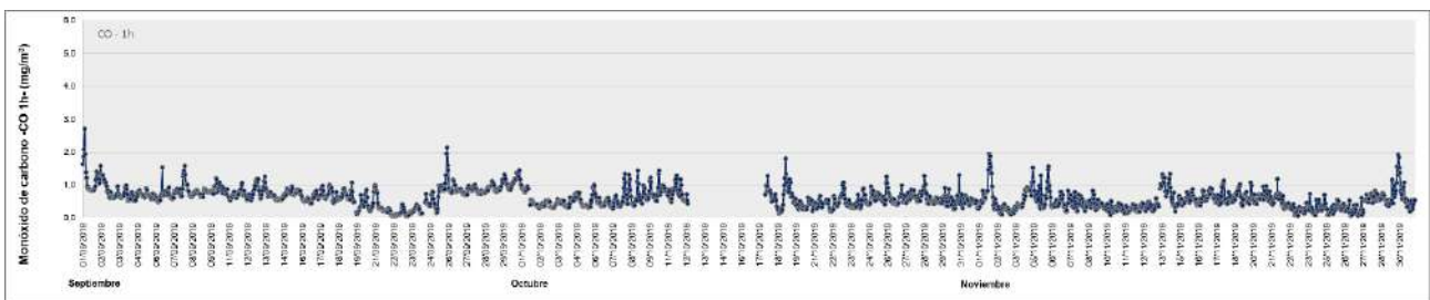
Figura 25. Variación horaria en la concentración de CO medida en la Estación de Monitoreo Continuo La Boca para el período septiembre - noviembre 2019. Los resultados se expresan en \text{mg}\cdot\text{m}^{-3} .
