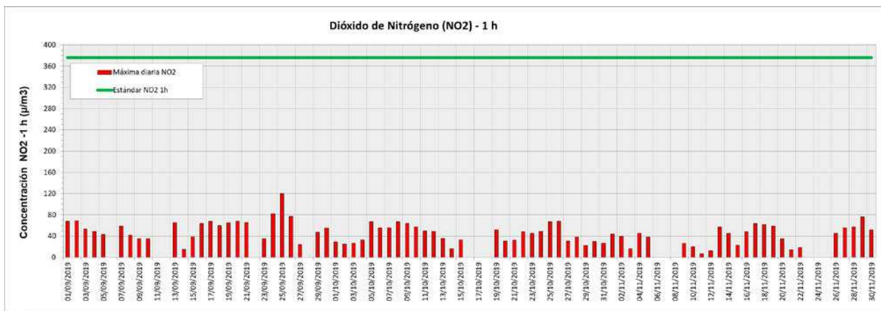
Figura 11. Valores de concentración máximos diarios de NO 2 (1 h) medidos en la Estación de Monitoreo Continuo Dock Sud (EMC I) período septiembre - noviembre 2019. Los resultados se expresan en µg.m -3 .
