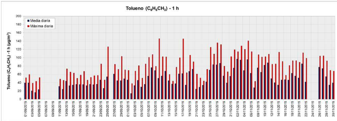
Figura 50. Valores de concentración medios y máximos diarios de tolueno (1 h) medidos en el equipo Open Path (OP2) ubicado en Dock Sud (período septiembre - noviembre 2019). Los resultados se expresan en \mu\text{g}\cdot\text{m}^{-3} .
