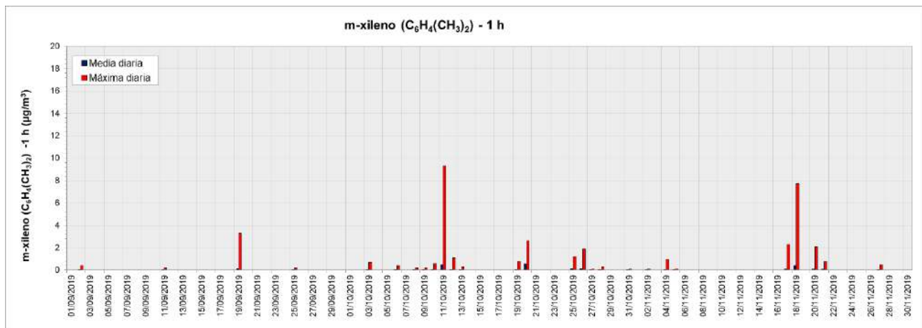
Figura 52. Valores de concentración medios y máximos diarios de m-Xileno (1 h) medidos en el equipo Open Path (OP2) ubicado en Dock Sud (período septiembre - noviembre 2019). Los resultados se expresan en \mu\text{g}\cdot\text{m}^{-3} .
