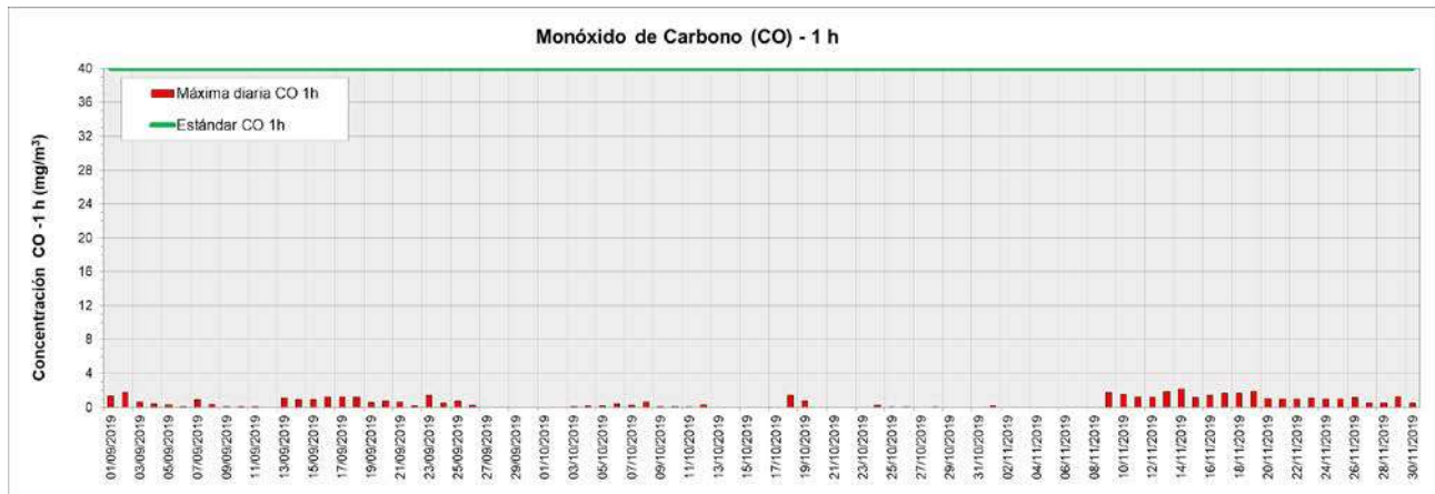
Figura 6. Valores de concentración máximos diarios de CO (1 h) medidos en la Estación de Monitoreo Continuo La Matanza (EMC II) período septiembre - noviembre 2019. Los resultados se expresan en \text{mg}\cdot\text{m}^{-3} .
