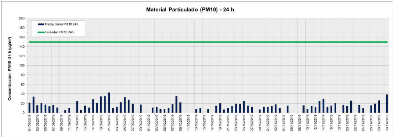
Figura 21. Valores de concentración medios de PM 10 (24 h) medidos en la Estación de Monitoreo Continuo La Matanza (EMC II) período septiembre - noviembre 2019. Los resultados se expresan en \mu\text{g}\cdot\text{m}^{-3} .
