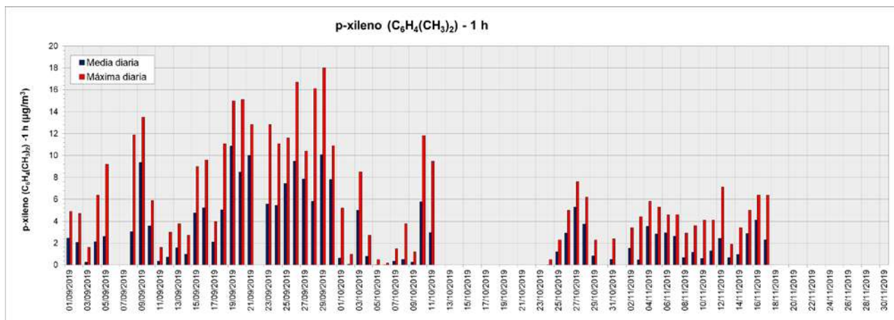
Figura 53. Valores de concentración medios y máximos diarios de p-Xileno (1 h) medidos en el equipo Open Path (OP1) ubicado en Dock Sud (período septiembre - noviembre 2019). Los resultados se expresan en µg.m -3 .
