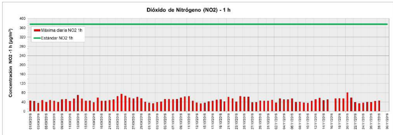
Figura 13. Valores de concentración máximos diarios de NO 2 (1 h) medidos en la Estación de Monitoreo Continuo La Boca período septiembre - noviembre 2019. Los resultados se expresan en µg.m -3 .
