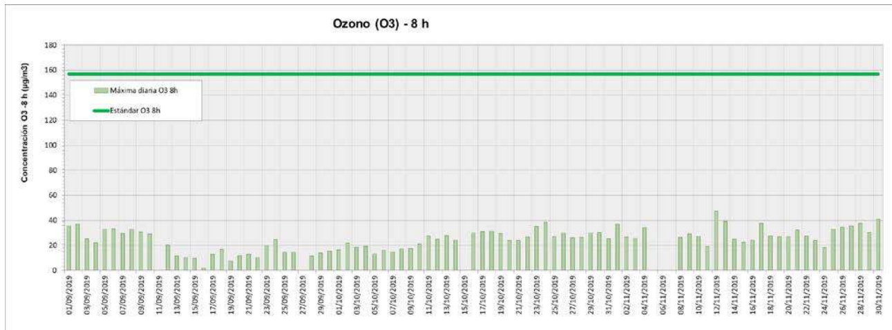
Figura 15. Valores de concentración máximos diarios de O 3 (8 h) medidos en la Estación de Monitoreo Continuo Dock Sud (EMC I) período septiembre - noviembre 2019. Los resultados se expresan en µg .m -3 .
