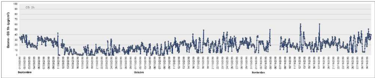
Figura 31. Variación horaria en la concentración de O 3 medida en la Estación de Monitoreo Continuo Dock Sud (EMC I) para el período septiembre - noviembre 2019. Los resultados se expresan en µg.m -3 .
