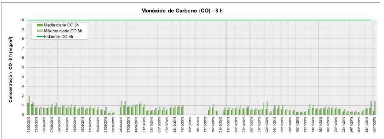
Figura 10. Valores de concentración máximos diarios de CO (8 h) medidos en la Estación de Monitoreo Continuo La Boca período septiembre - noviembre 2019. Los resultados se expresan en \text{mg}\cdot\text{m}^{-3} .
