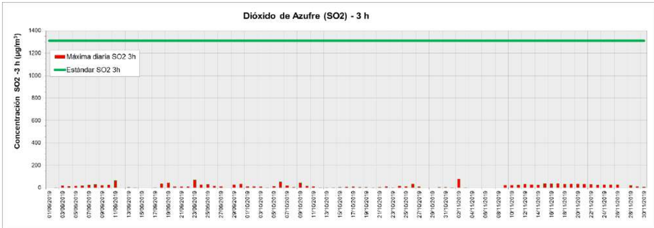
Figura 17. Valores de concentración máximos diarios de SO 2 (3 h) medidos en la Estación de Monitoreo Continuo La Matanza (EMC II) período septiembre - noviembre 2019. Los resultados se expresan en µg.m -3 .
