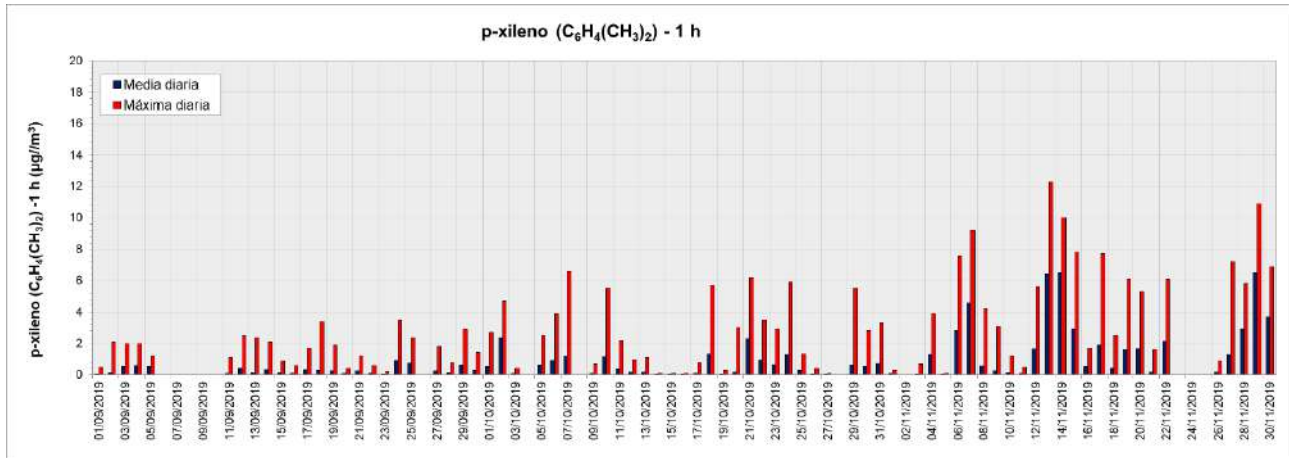
Figura 54. Valores de concentración medios y máximos diarios de p-Xileno (1 h) medidos en el equipo Open Path (OP2) ubicado en Dock Sud (período septiembre - noviembre 2019). Los resultados se expresan en \mu\text{g}\cdot\text{m}^{-3} .
