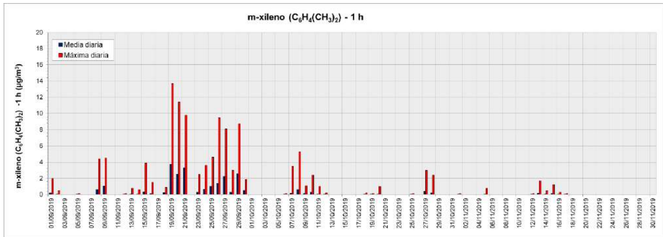
Figura 51. Valores de concentración medios y máximos diarios de m-xileno (1 h) medidos en el equipo Open Path (OP1) ubicado en Dock Sud (período septiembre - noviembre 2019). Los resultados se expresan en \mu\text{g}\cdot\text{m}^{-3} .
